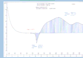
Fig 4. Oxyma Pure
