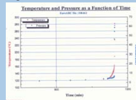
Fig 7. Oxyma Pure
